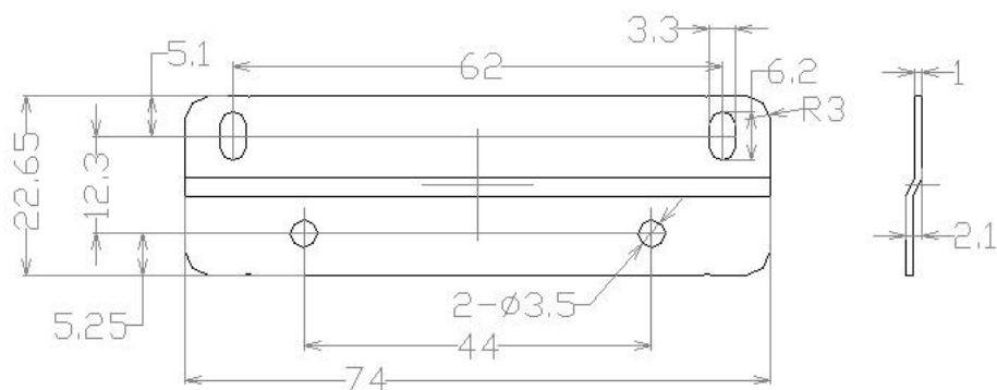
固定片尺寸
