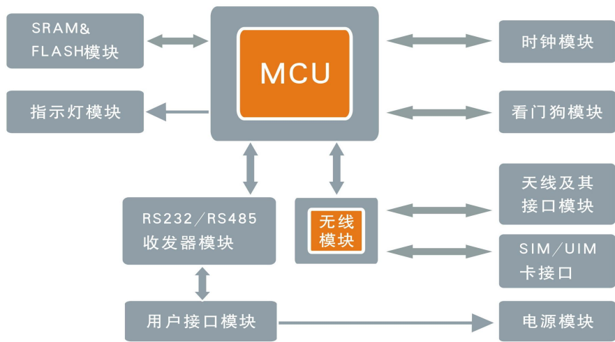
图 1-2 IP MODEM 结构框图
